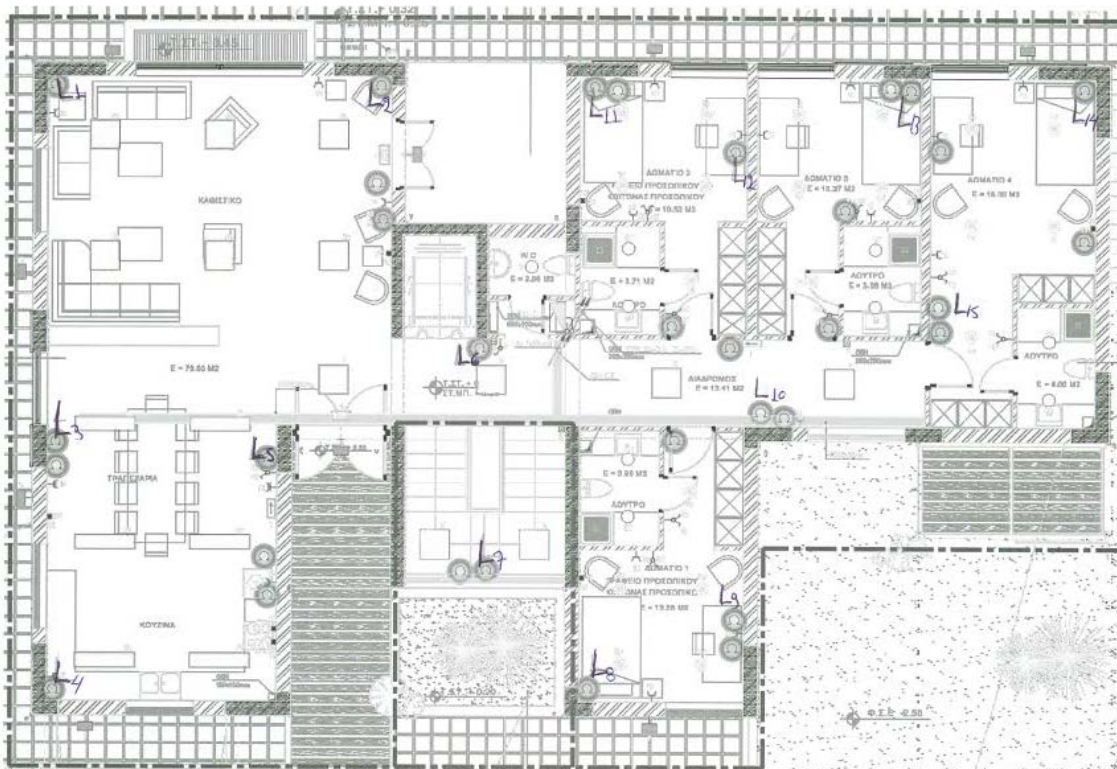
Εικόνα 1: Κάτοψη ισογείου τέταρτης ΣΥΔ
